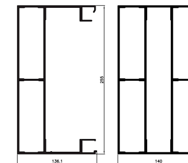
Subgrinda extremă și intermediară cu dimensiunile 140×255 mm
